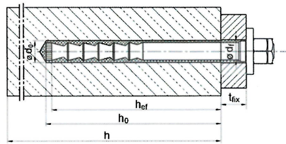
Durchsteckmontage
