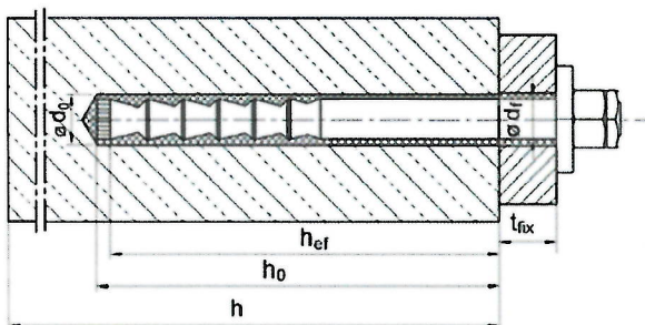
Vorsteckmontage
