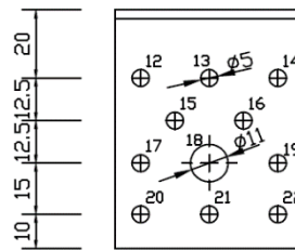
Abbildung A.2 Abmessungen des Winkelverbinders 70 ohne Steg
