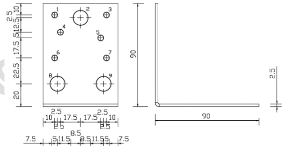
Abbildung A.4 Abmessungen des Winkelverbinders 90 ohne Steg
