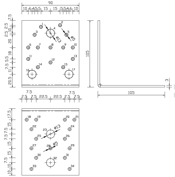
Abbildung A.6 Abmessungen des Winkelverbinders 105 ohne Steg
