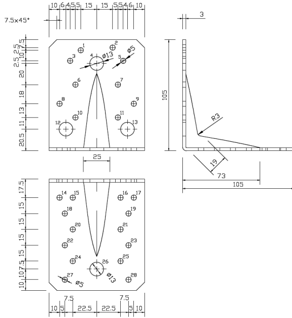
Abbildung A.5 Abmessungen des Winkelverbinders 105 mit Steg
