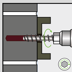
4. Einschrauben (Bohrschrauber)
