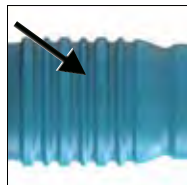
Doppel-Dichtlippe Für optimale Ab- dichtung zwischen Dübel und Baustoff, ohne den Einsatz von Silikon.
