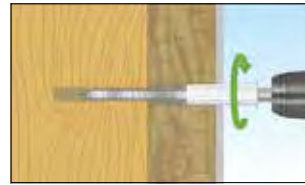
Fertig eindrehen bis der Kragen des Entkopplungselements bündig am Putz anliegt.
