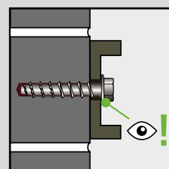
5. Kopfaufgabe beachten → Fertig.
