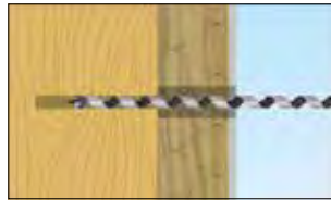
Bohrloch mit \varnothing 5 mm im Holz erstellen. Bohrlochtiefe: \geq 30 mm + t_{WDVS}
