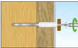
3.2 Befestigung des Anbauteils mit einer Schraube \varnothing 3,0 - 4,5.
