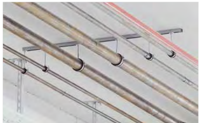
Rohrmontage
